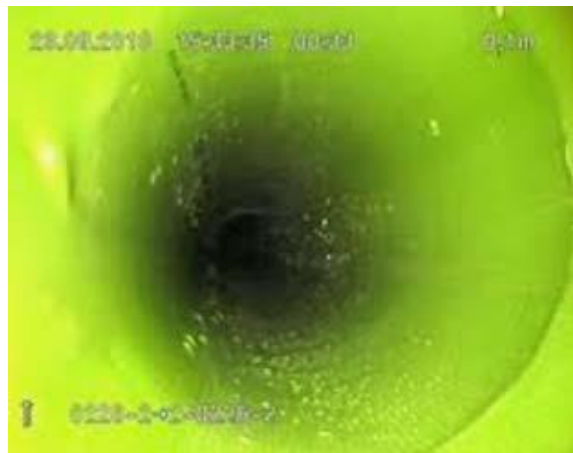
Schmutzwasserkanal nach Einbau des Schlauchliners
