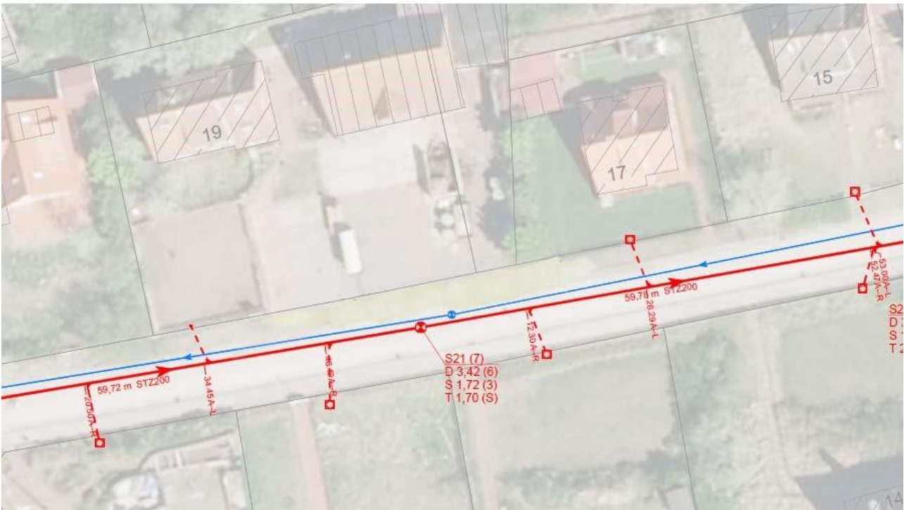
Abbildung: Beispiel für eine Trennkanalisation mit Darstellung der Schmutzwasserkanalisation einschließlich Anschlusskanal Hausrevisionsschacht (Darstellung in rot)
